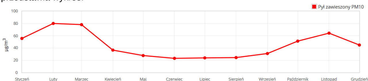
Rysunek 7 Wyniki badań powietrza uzyskane na stacji przy ul. Skłodowskiej w 2018 roku dla pyłu zawieszonego PM10
