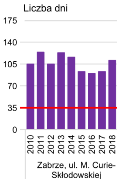
Rysunek 6 Liczba dni z przekroczeniem stężeń dobowych pyłu PM10 powyżej 50 µg/m³ w aglomeracji górnośląskiej w latach 2010-2018
