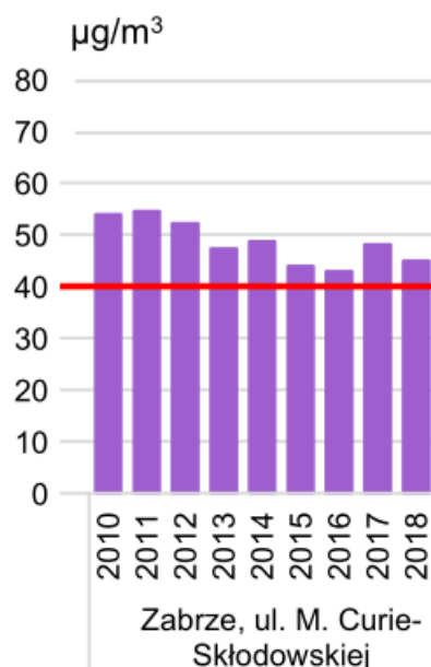
Rysunek 5 Stężenia średnie roczne pyłu PM10 w aglomeracji górnośląskiej w latach 2010-2018
