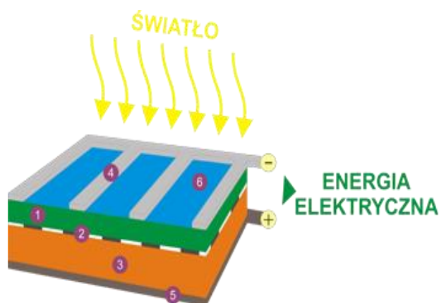
Rysunek 1 Budowa ogniwa fotowoltaicznego
