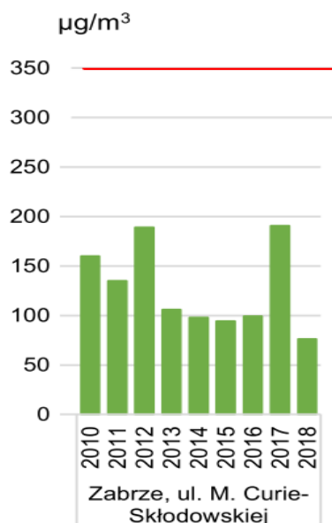
Rysunek 3 Stężenia 1-godzinne dwutlenku siarki (25 maksymalne) w aglomeracji górnośląskiej w latach 2010-2018 (poziom dopuszczalny stężenia 1-godz. 350 µg/m³)
